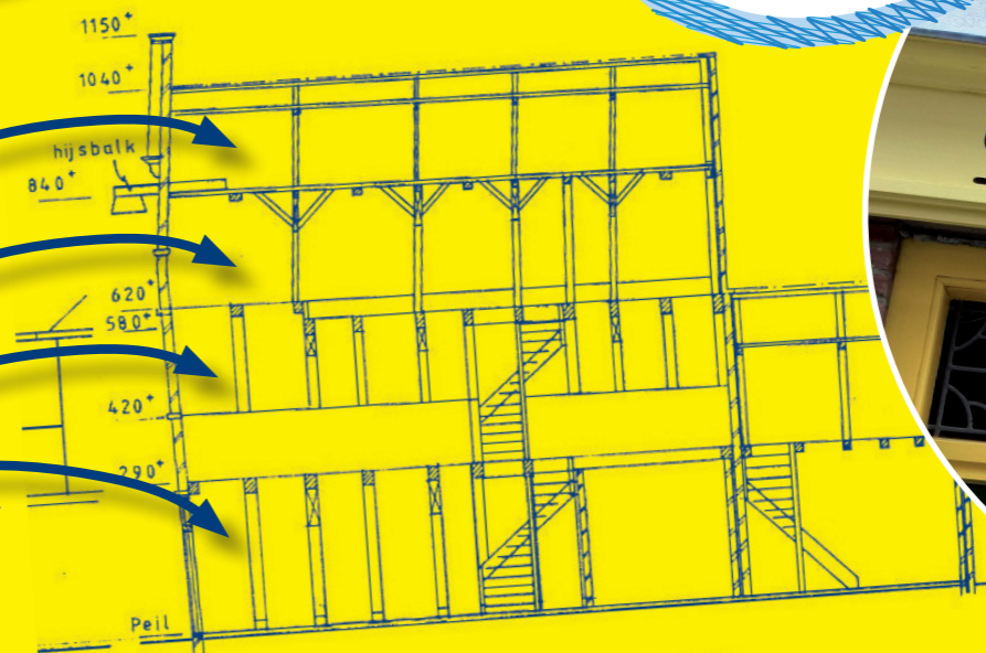
langsdoorsnede
